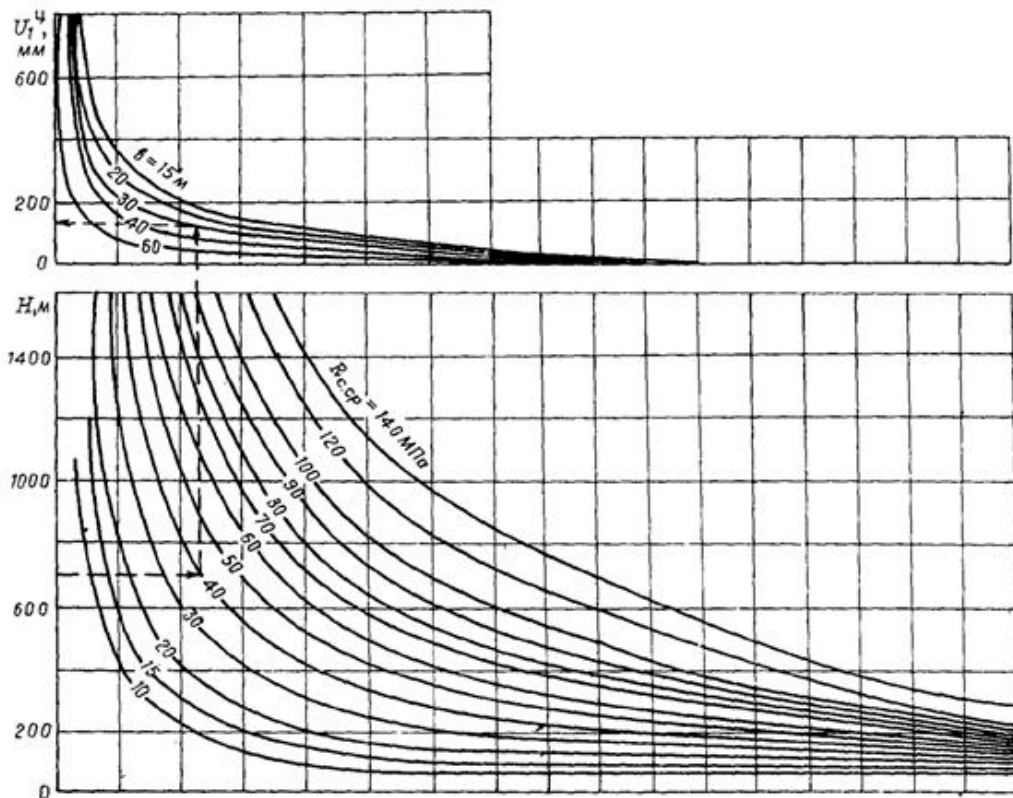
Рис. 9. Номограмма для определения U_1^{II}
