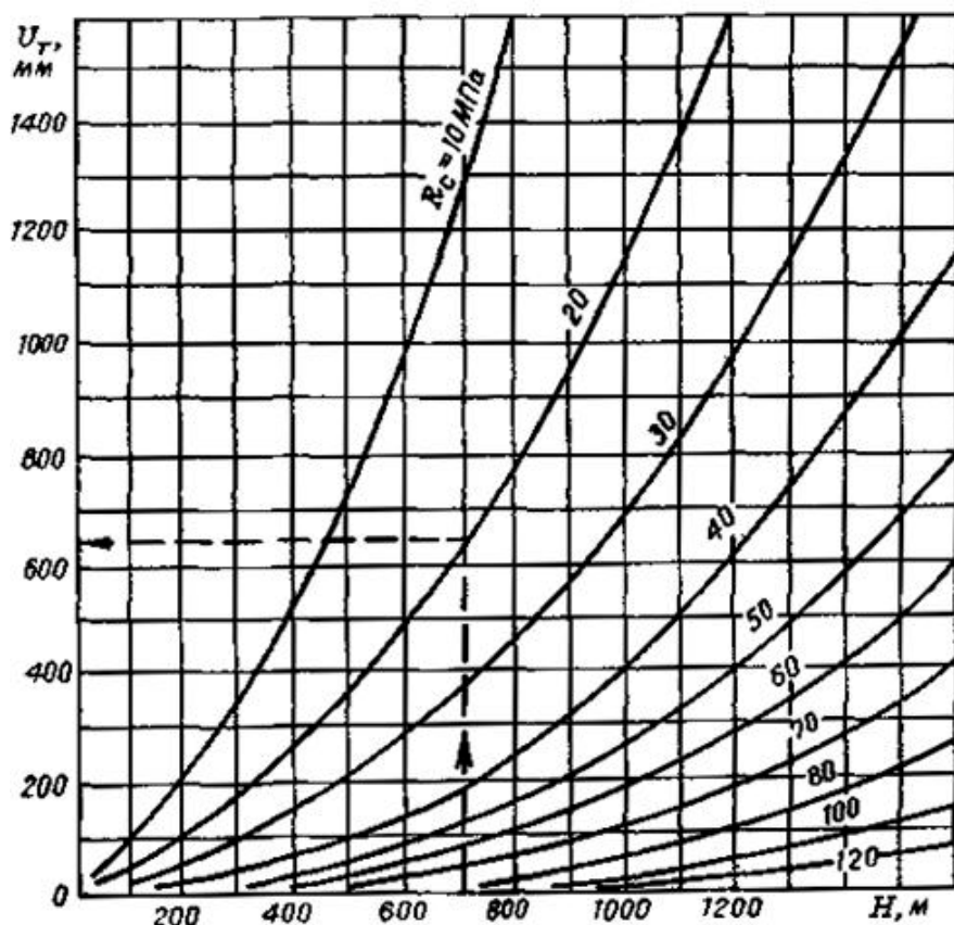
Рис. 2. Графики для определения типического смещения пород
